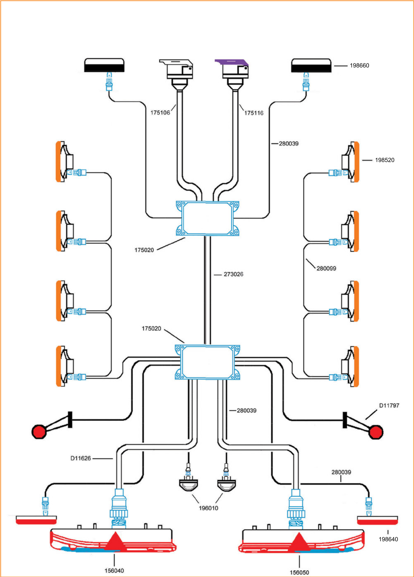
Exemple de montage - Esempio di montaggio - Ejemplo de montaje
