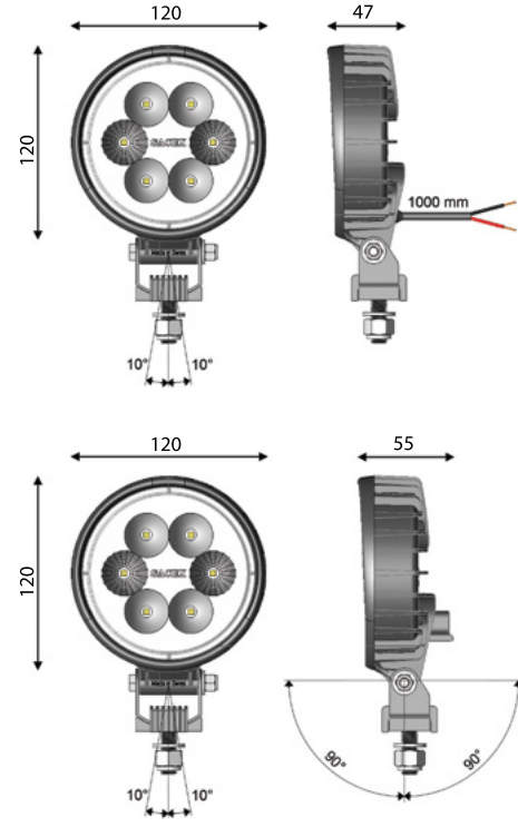
DT 2 voies - 2 vie - 2 vías
