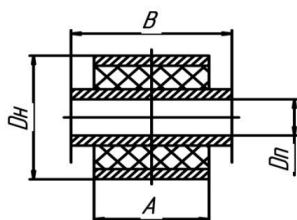
Сайлентблок:
