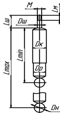
Тип 3: штырь-проушина
