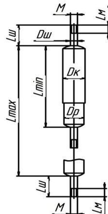
Тип 4: штырь-штырь
