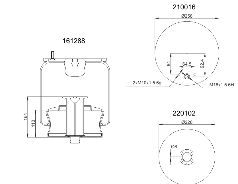
(Steel Piston)
